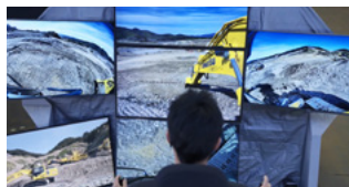
遠隔操作ポッドによる油圧ショベル「PC200i-11」の遠隔操作(石川県)
